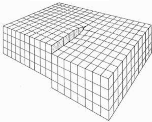
Figure: 5 Edge Dislocation
